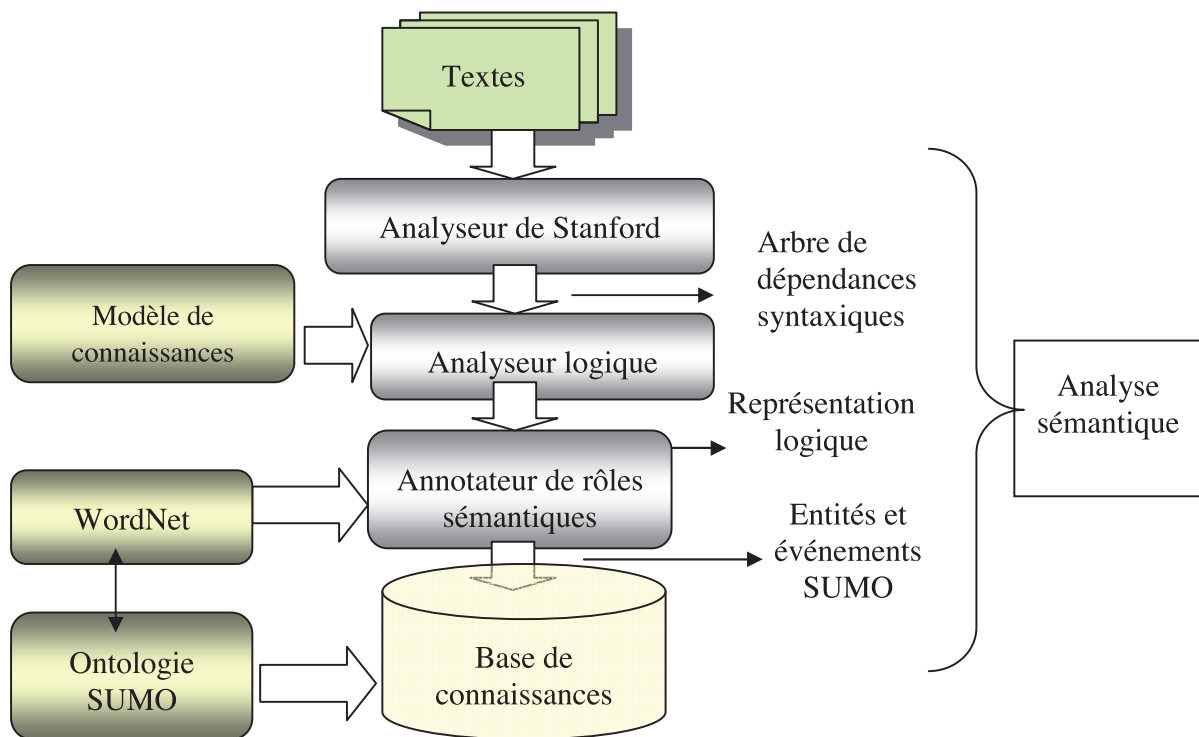
Figure 1 : Architecture modulaire pour l'analyse sémantique
