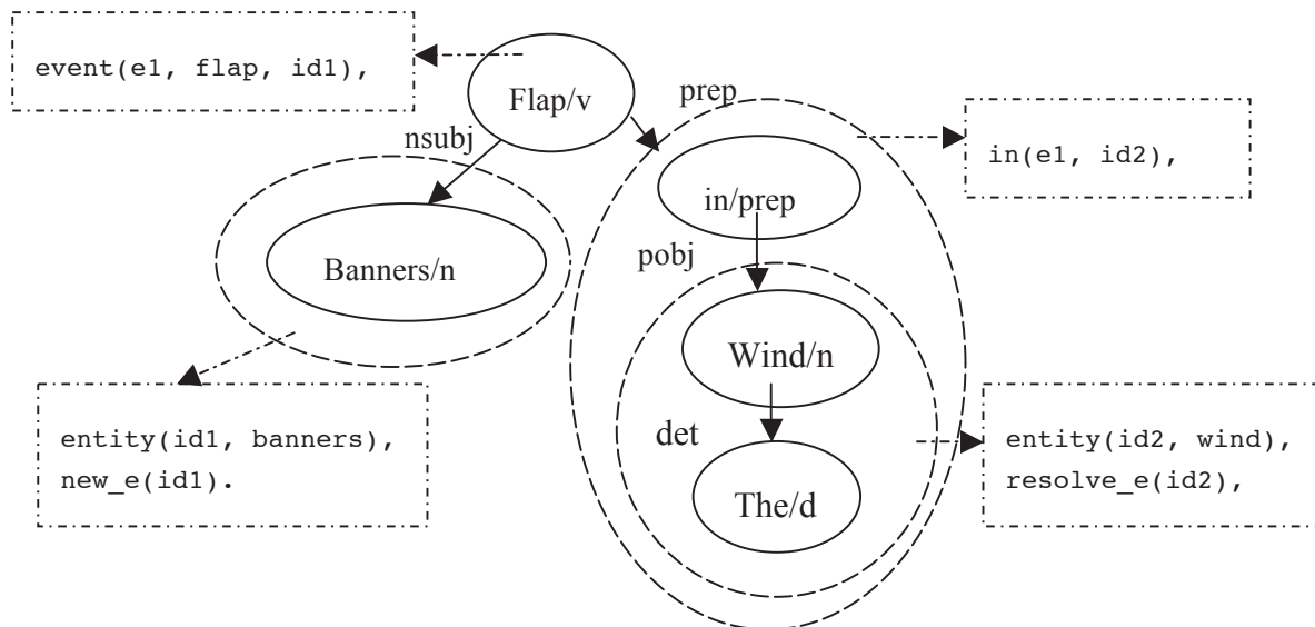
Figure 2: Un exemple des différentes sous-analyses compositionnelles
