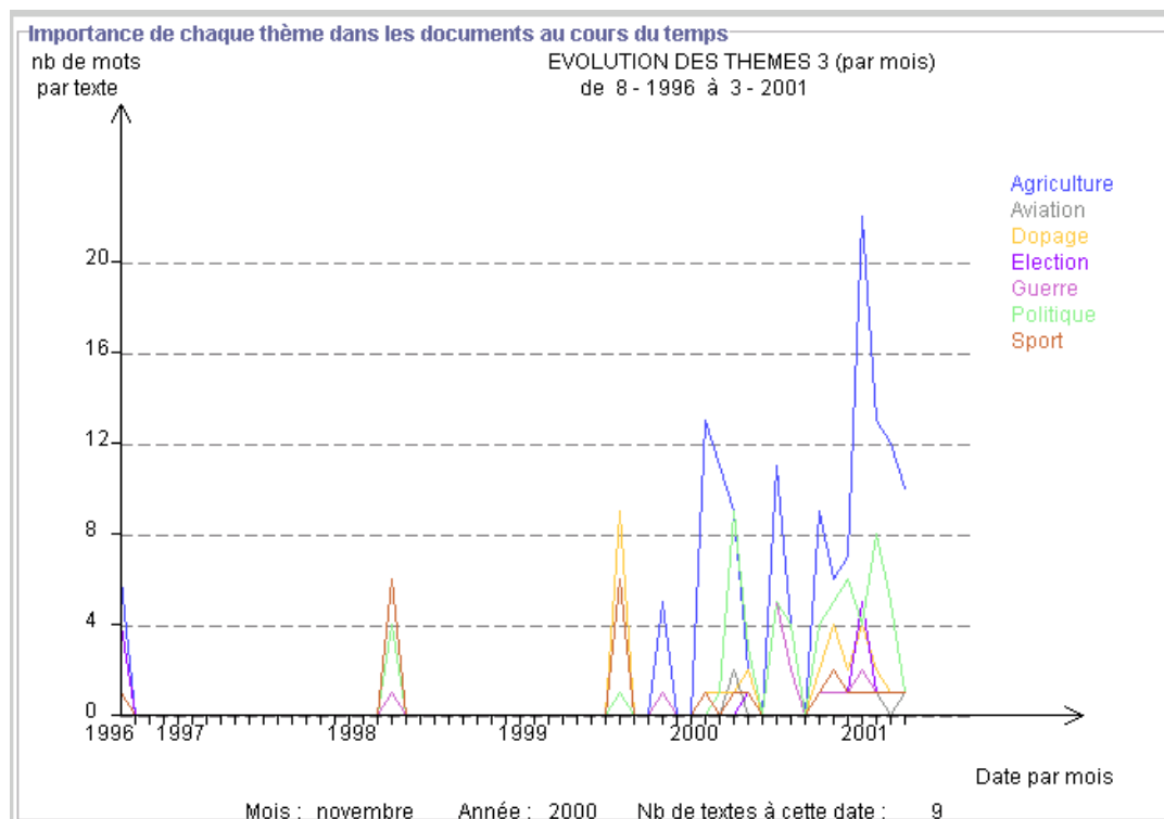
Figure 9 : Analyse de l'évolution des thèmes dans un flux documentaire
