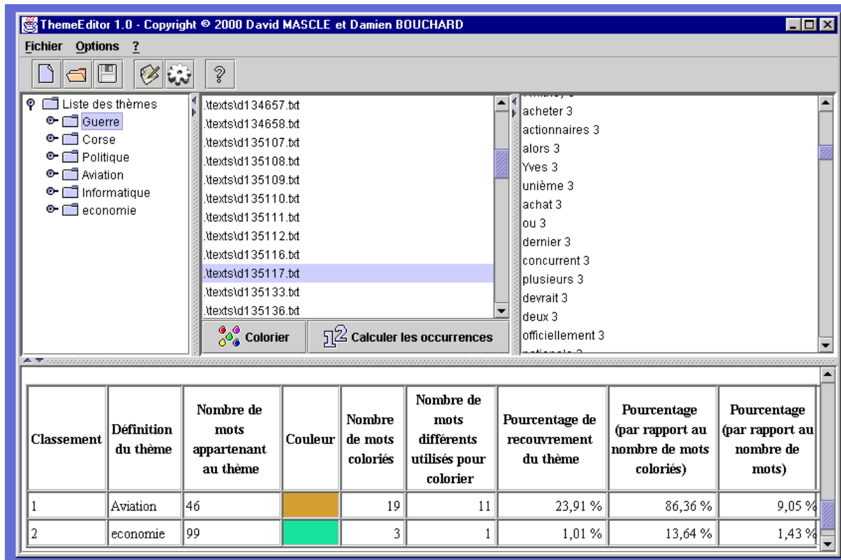
Figure 3 : L'interface de ThemeEditor : Résultats statistiques du coloriage du texte d135117.txt
