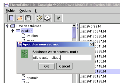
Figure 4. Saisie d'une lexie au clavier : ajout de « pilote automatique » dans le thème aviation.
